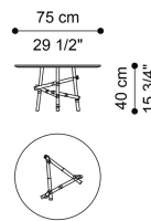
LOW TABLE E.SAM.232.A
