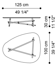
LOW TABLE E.SAM.231.A
