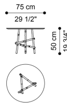
LOW TABLE E.SAM.232.C
